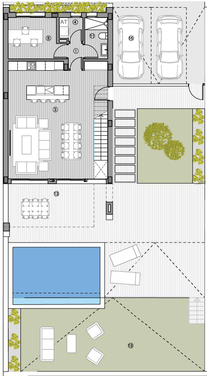
PLANTA BAJA
